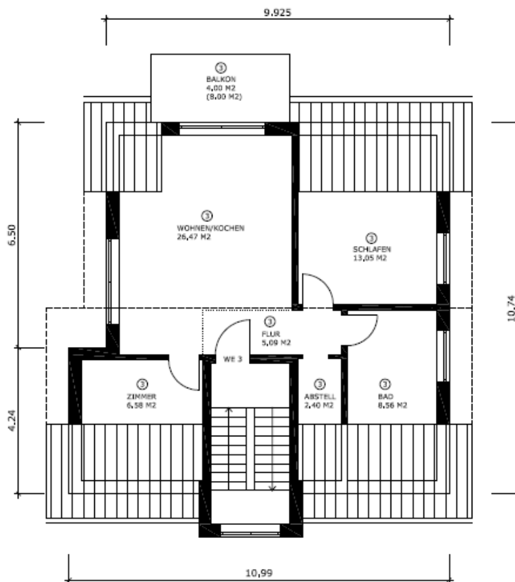
GRUNDRISS DG
